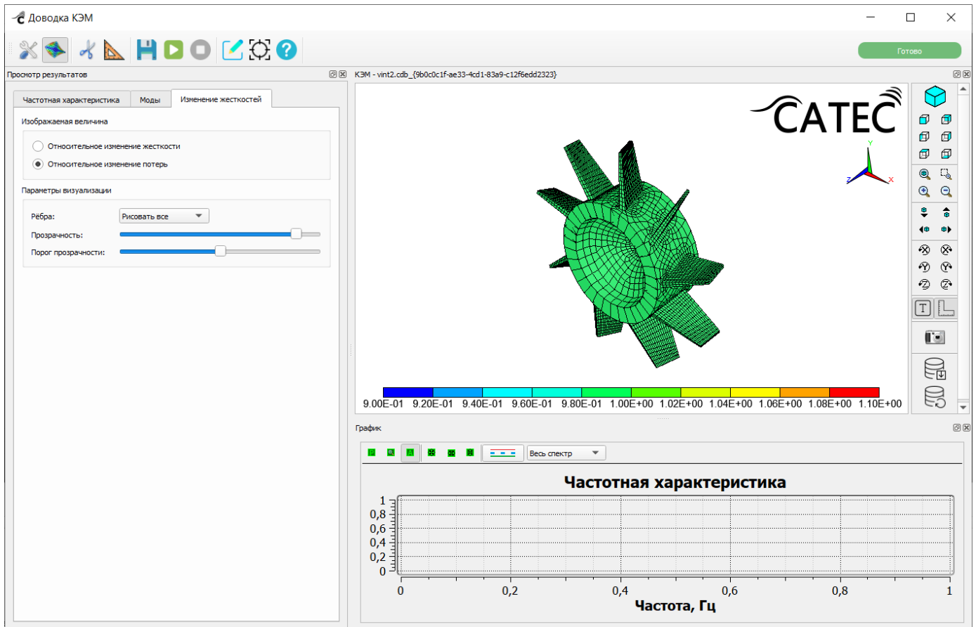
Рисунок 339 – Изображение относительного изменения упругости в элементах суперэлемента в модуле «Доводка КЭМ»
