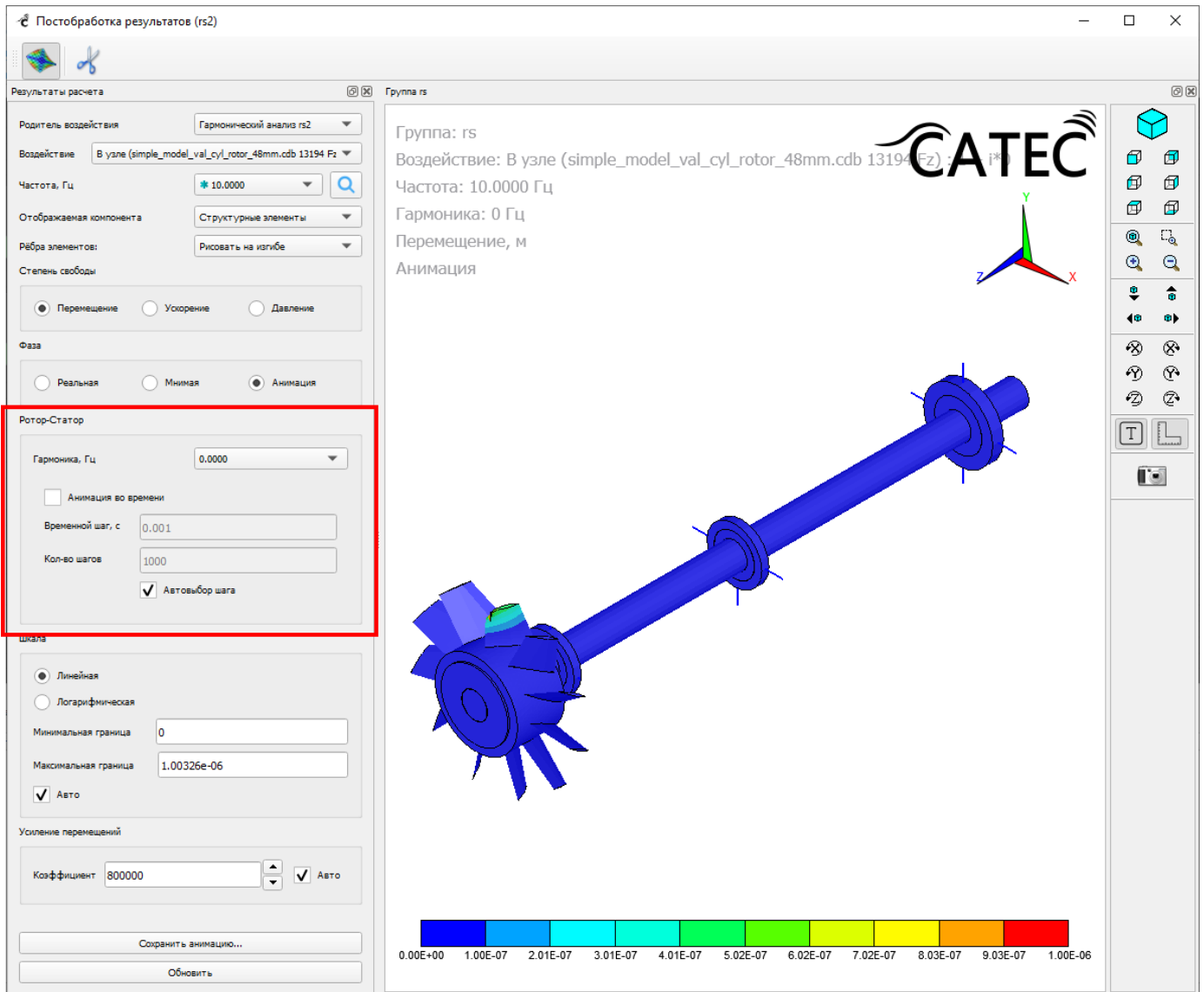
Рисунок 320 – Параметры интерфейса «Ротор-Статор»
