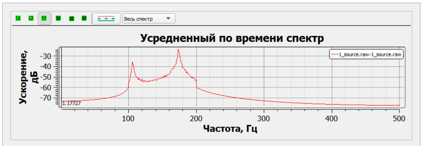
Рисунок 366 – Усредненный по времени спектр сигнала для двух каналов
