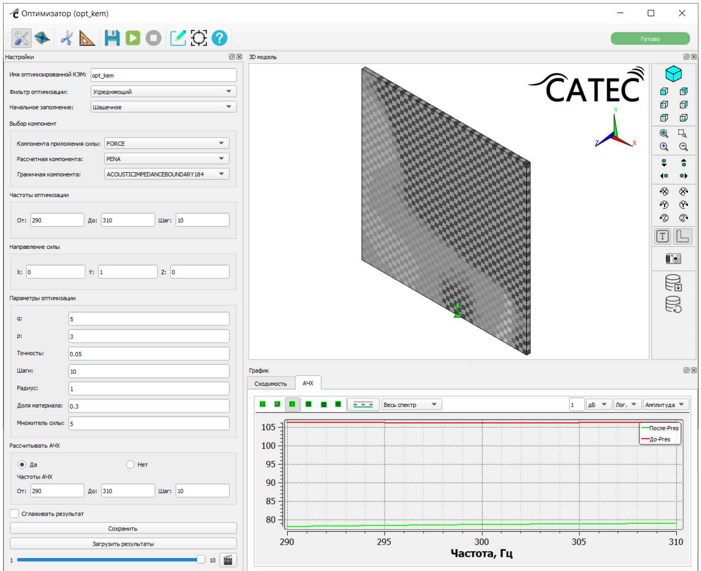
Рисунок 153 – Оптимизированная КЭМ. График АЧХ
