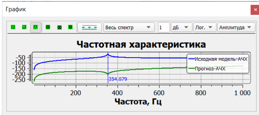
Рисунок 336 – Пример графика АЧХ исходной модели с указанием и прогноза АЧХ выбранной частоты (354.079 Гц на графике) в модуле «Доводка КЭМ»
