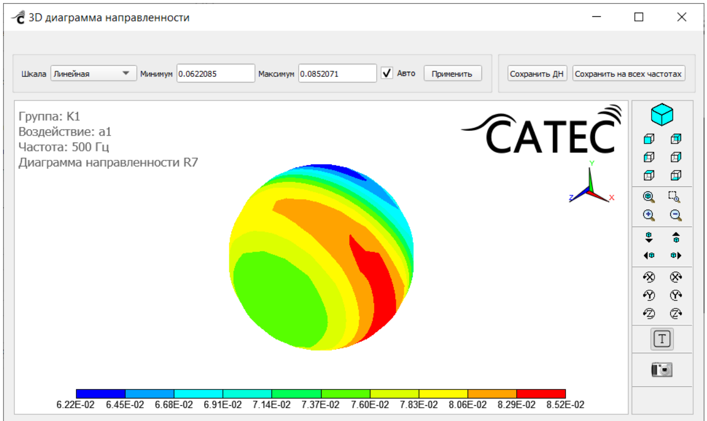
Рисунок 311 – Построение рассчитанных диаграмм направленности
