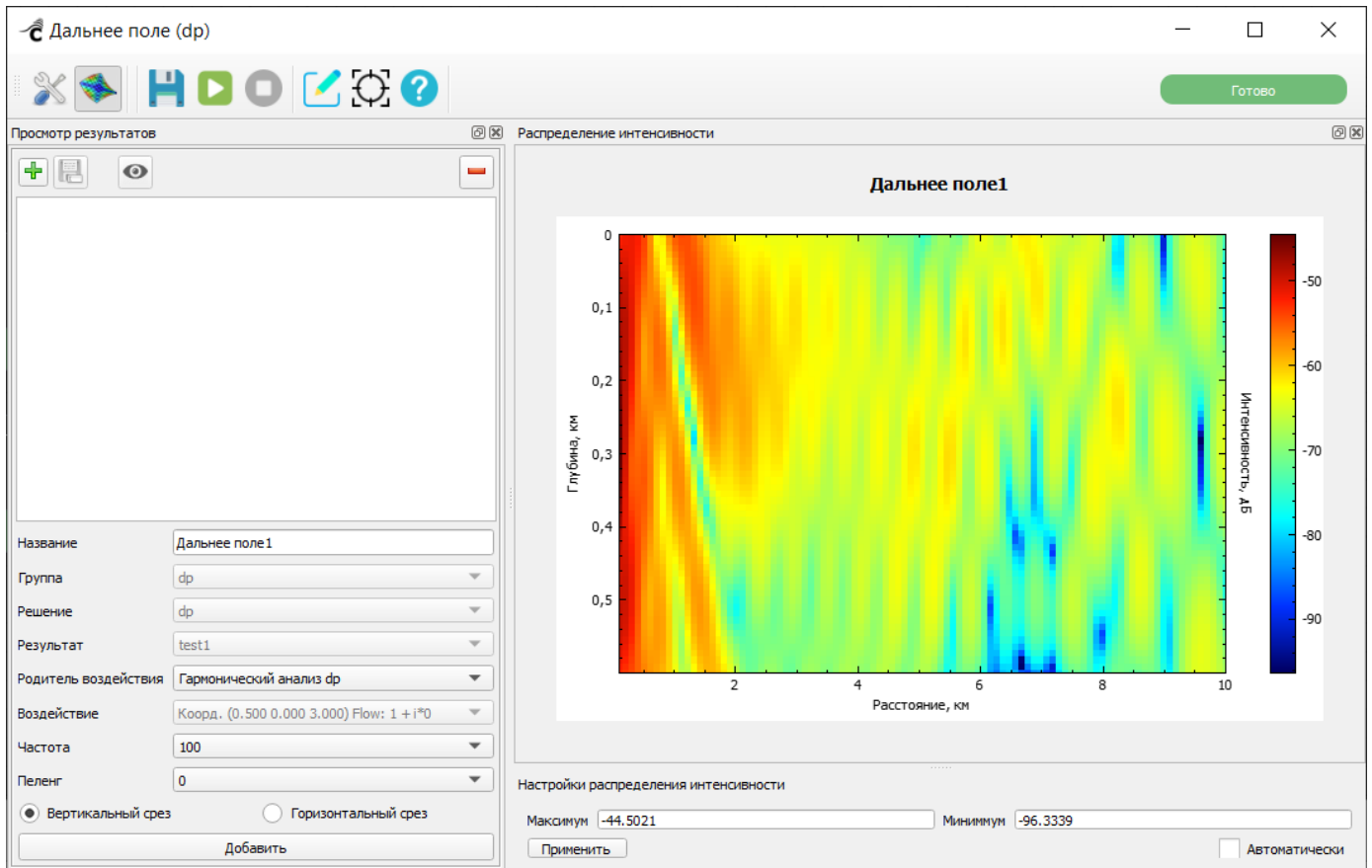
Рисунок 226 – График распределения интенсивности дальнего поля при вертикальном срезе
