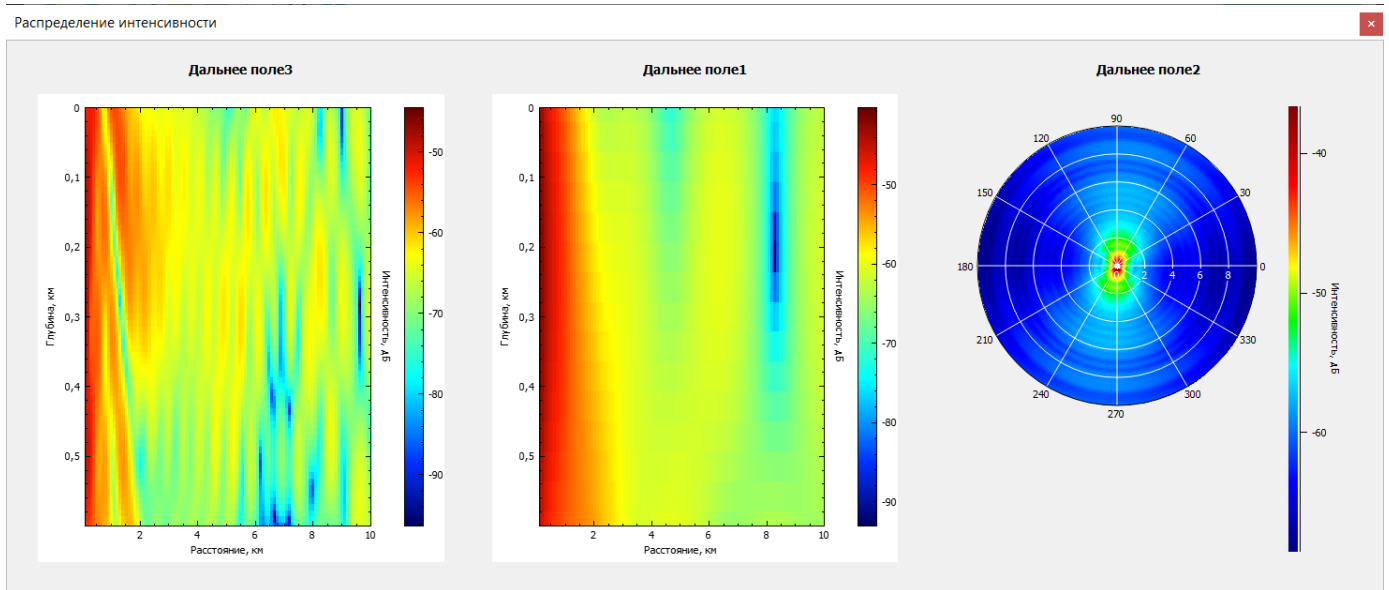
Рисунок 228 – Пример сравнения графиков распределения интенсивности в постобработке результатов карточки «Дальнее поле». Окно «Распределение интенсивности» в свободном состоянии, сравниваются 4 графика
