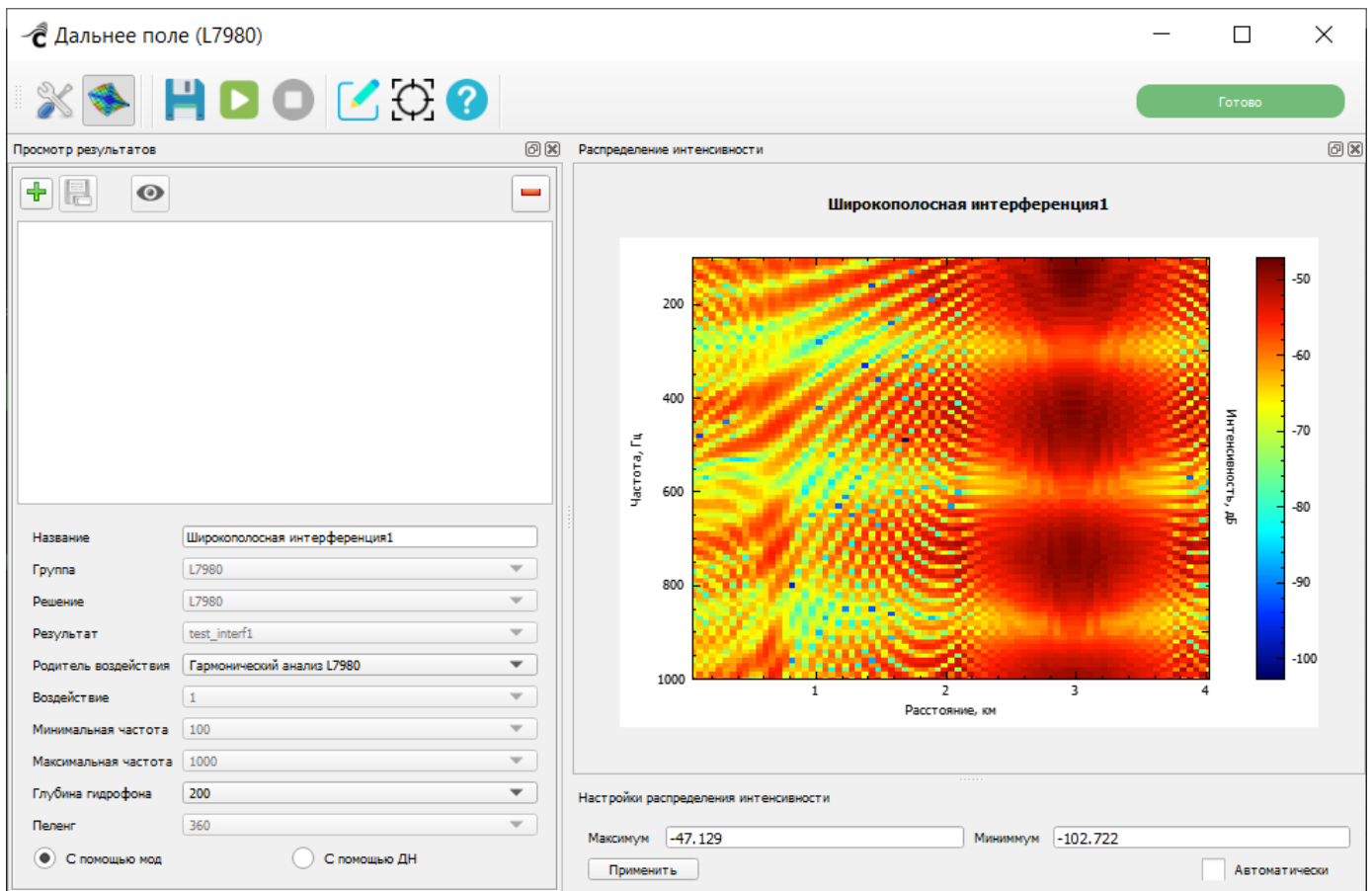
Рисунок 230 – График широкополосной интерференции, рассчитанный методом нормальных мод
