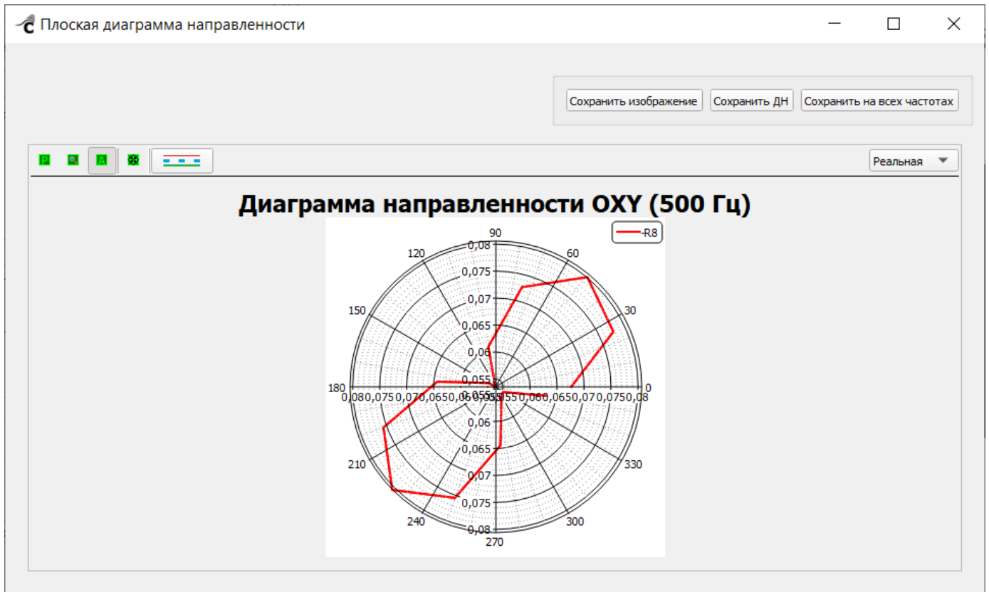
Рисунок 315 – Отображение плоской диаграммы направленности
