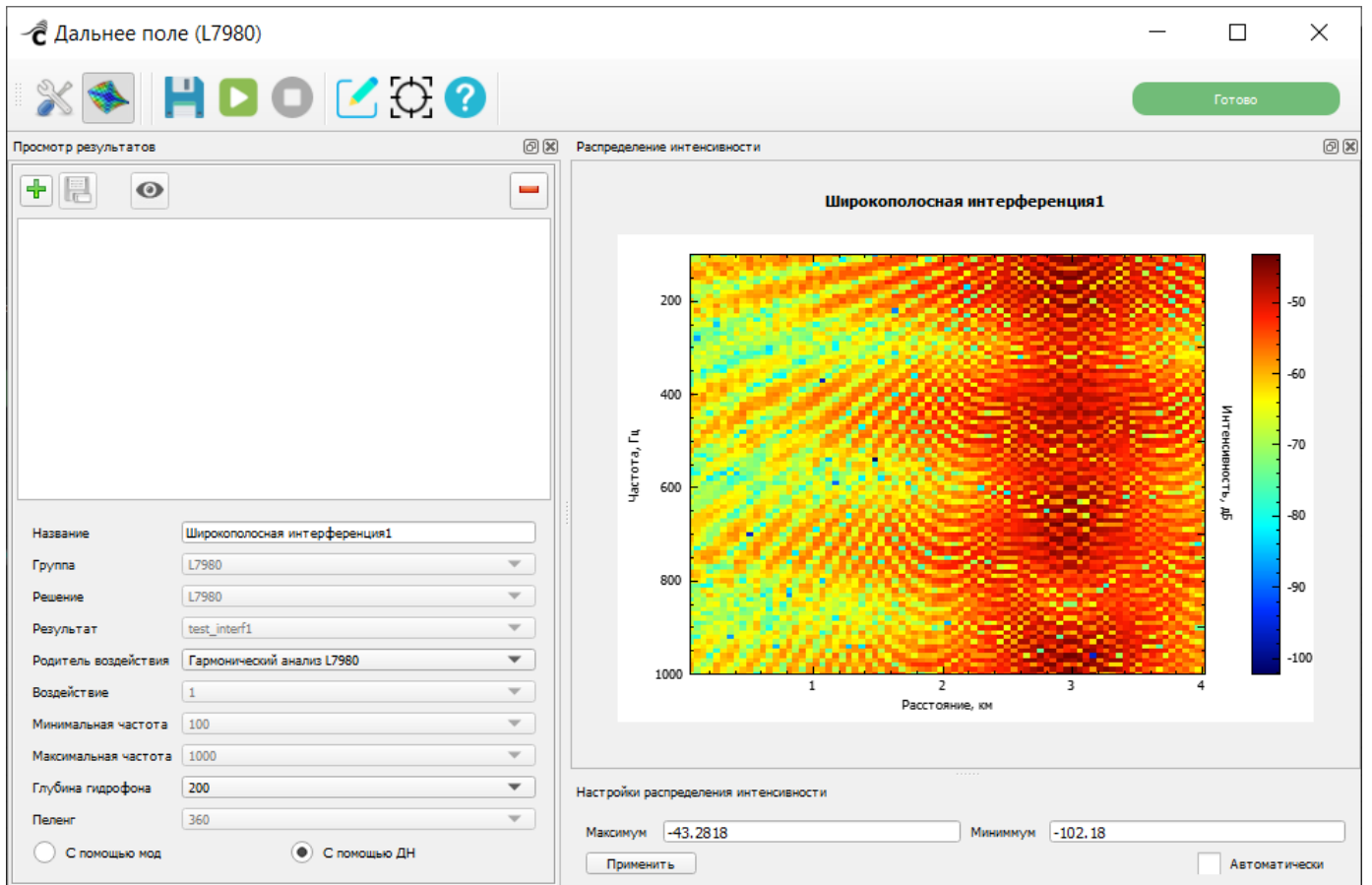
Рисунок 231 – График широкополосной интерференции, рассчитанный методом мнимых источников
